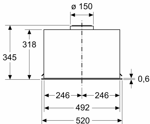
Méretetek mm-ben
