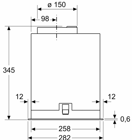
Méretetek mm-ben
