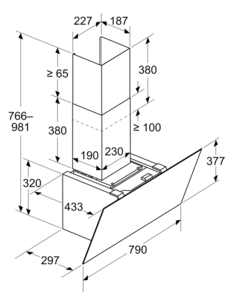
Méretetek mm-ben Készülék légkivezetéses üzemmódban
