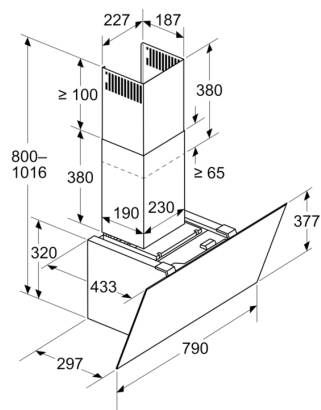
Méreték mm-ben Készülék levegőkeringetési üzemmódban
