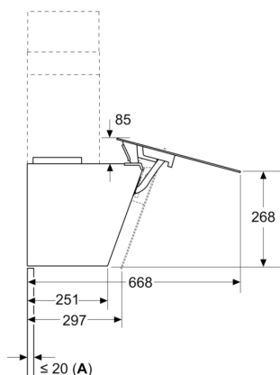
Méretetek mm-ben
