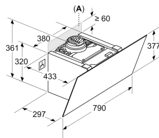
Méreték mm-ben Készülék levegőkeringetési üzemmódban csatorna nélkül
