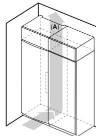
A: Légkivezető \geq 200 \text{ cm}^2
