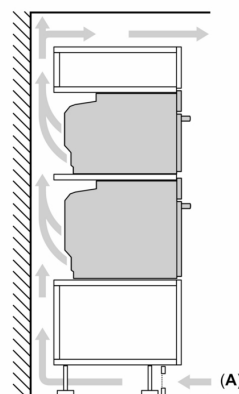
Két készülék beépítése egymás fölé Levegőcsere
